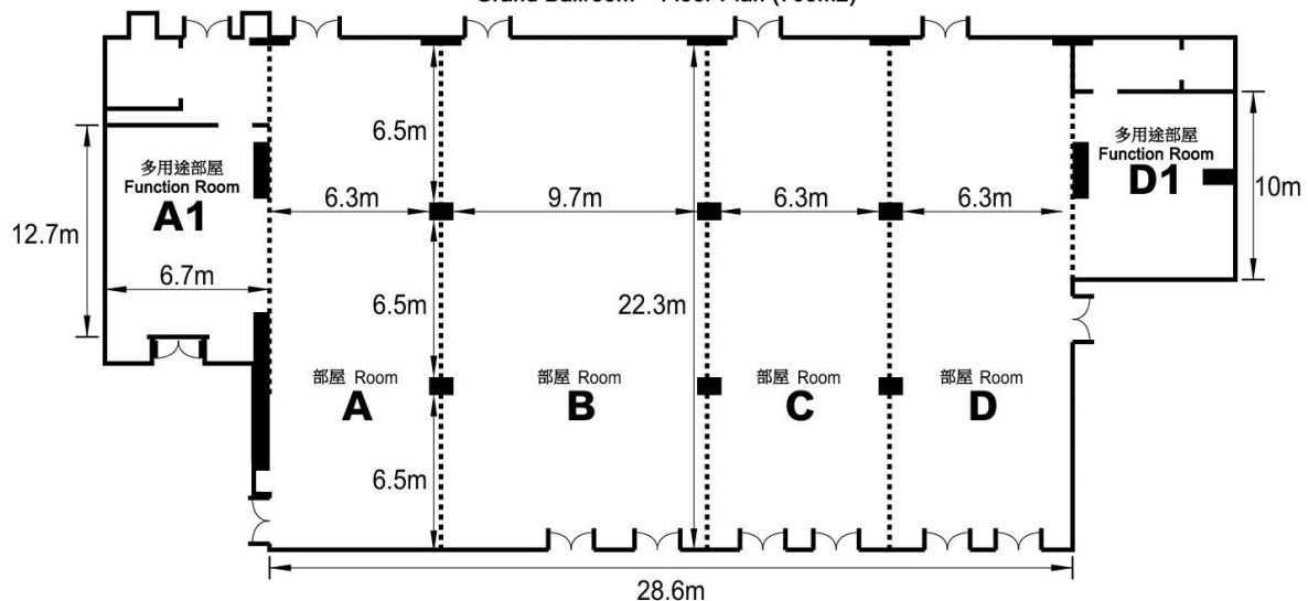
宴会ホール-平面図 (700平方米) Grand Ballroom - Floor Plan (700m 2 )
